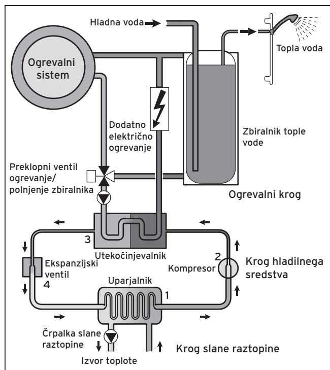
Sl. 3.4 Način delovanja toplotne črpalke (notranja enota)
