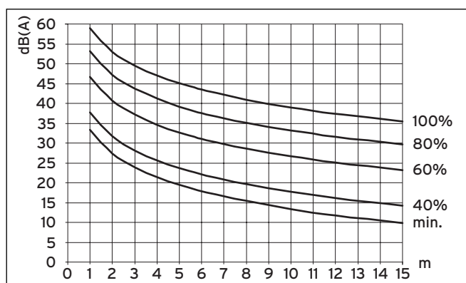
Sl. 6.5 Nivo zvočnega tlaka zunanje enote v dB(A) v odvisnosti od oddaljenosti in števila vrtljajev ventilatorja za VWL 171/3 S pri namestitvi na prostem
