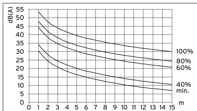
Sl. 6.2 Nivo zvočnega tlaka zunanje enote v dB(A) v odvisnosti od oddaljenosti in števila vrtljajev ventilatorja za VWL 81/3 S pri namestitvi na prostem
