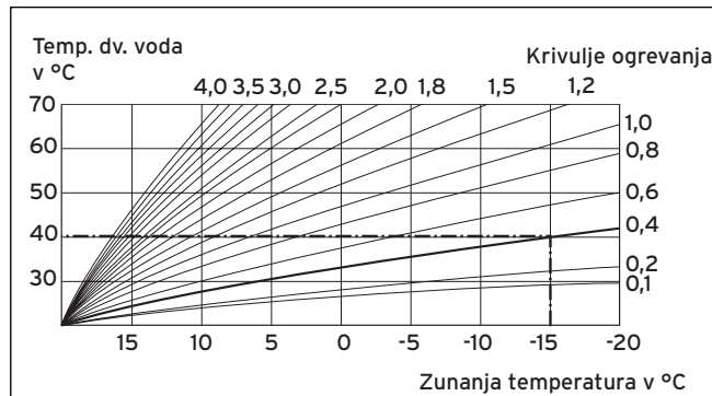
Sl. 1 Diagram krivulj ogrevanja
