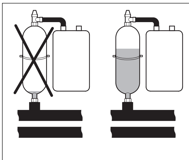
Sl. 6.5 Nivo napolnjenosti izravnalne posode za slano raztopino
