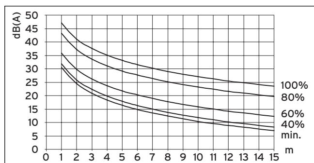
Sl. 6.1 Nivo zvočnega tlaka zunanje enote v dB(A) v odvisnosti od oddaljenosti in števila vrtljajev ventilatorja za VWL 61/3 S pri namestitvi na prostem
